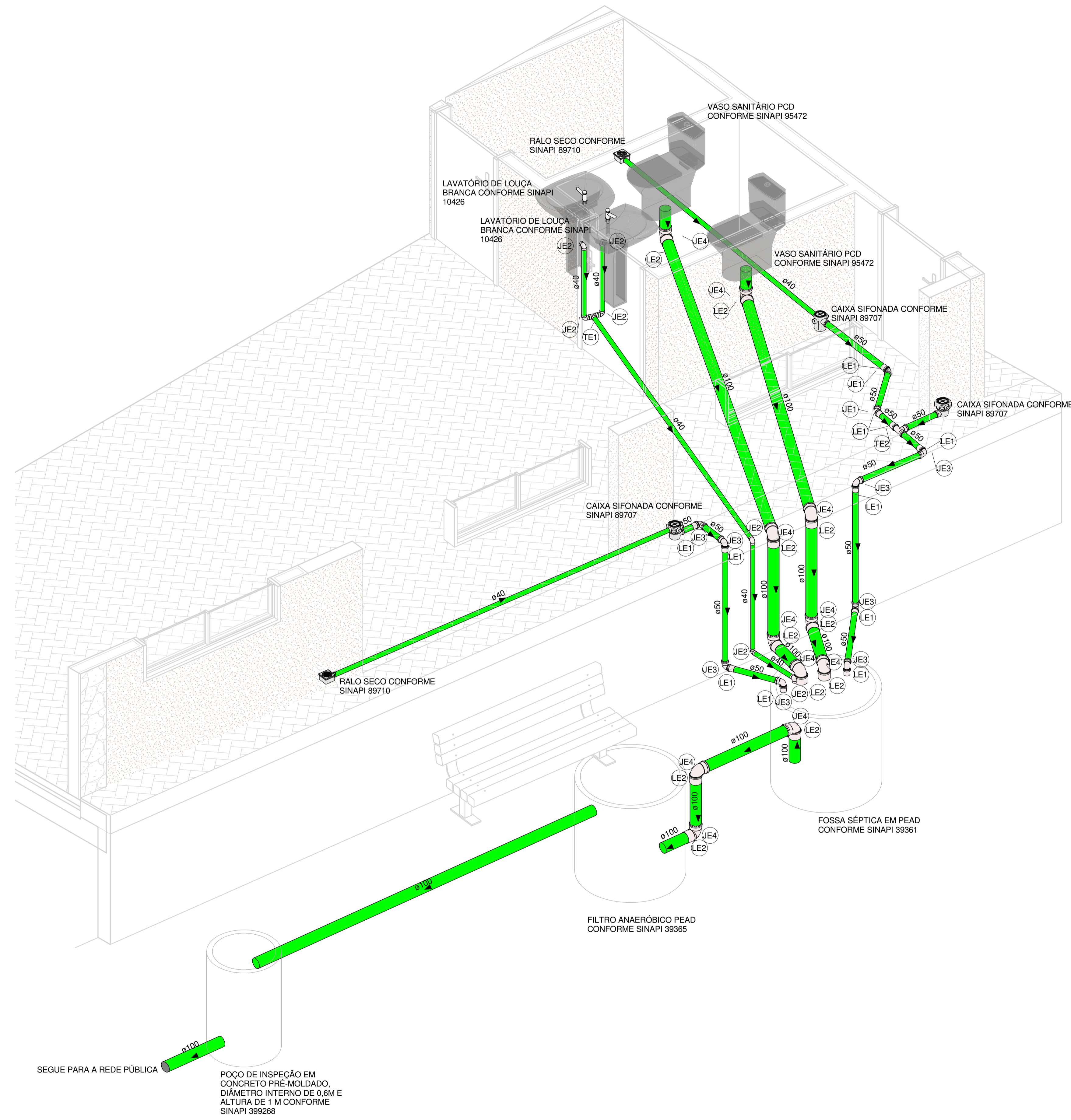
1 ISOMÉTRICO - SANITÁRIO
